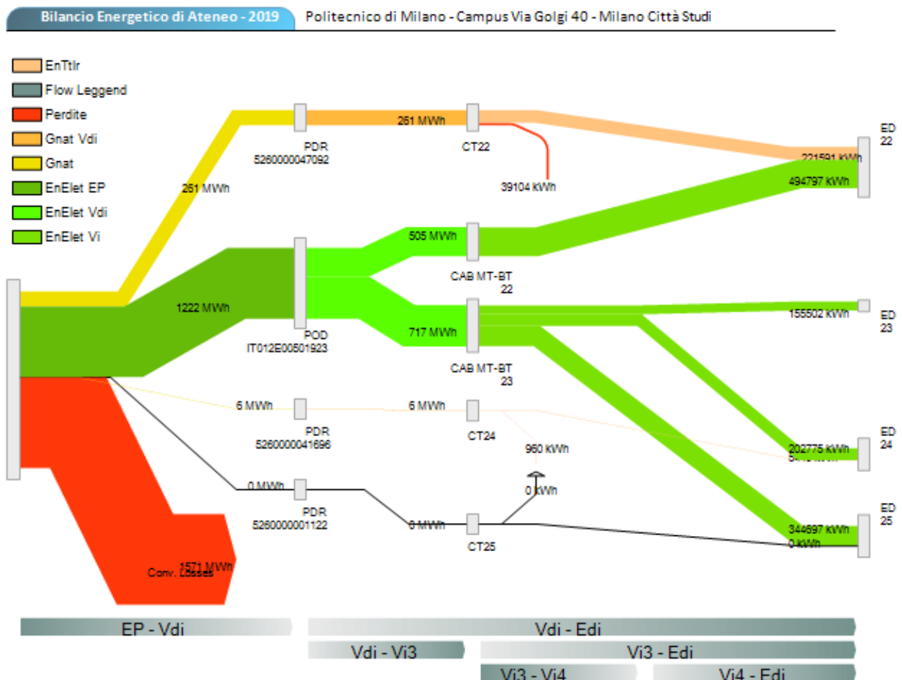
Figura 24. Diagramma di flusso dei vettori energetici, Campus via Golgi 40
