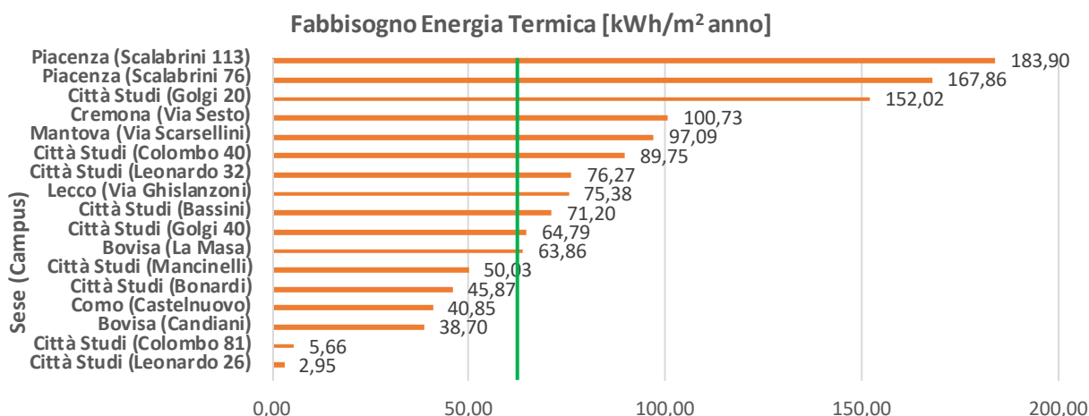
Figura 120. KPI calcolati fabbisogno energia termica a livello di Campus
