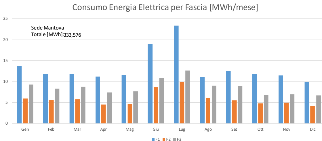
Figura 71. Consumo mensile energia elettrica suddiviso nelle fasce F1, F2, F3, Sede Mantova
