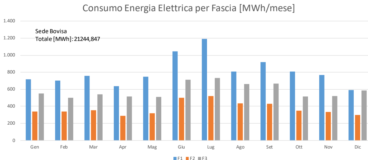
Figura 32. Consumo mensile energia elettrica suddiviso nelle fasce F1, F2, F3, Sede Milano Bovisa
