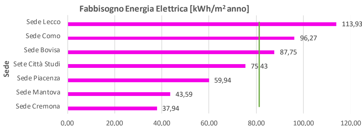
Figura 117. KPI calcolati fabbisogno energia elettrica a livello di Sede
