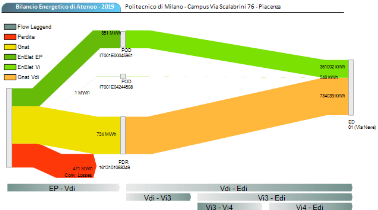
Figura 87. Diagramma di flusso dei vettori energetici, Campus Via Scalabrini 76
