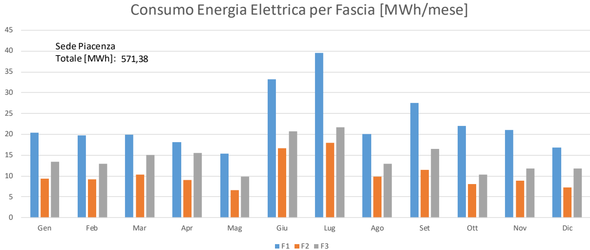
Figura 78. Consumo mensile energia elettrica suddiviso nelle fasce F1, F2, F3, Sede Piacenza
