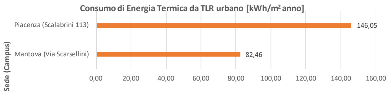
Figura 116. KPI consumo Energia Termica a livello di Campus
