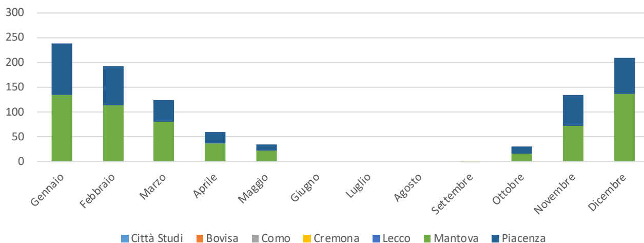
Figura 10. Consumo mensile da TLR esterno [MWh] anno 2019 suddiviso per due Sedi del Politecnico
