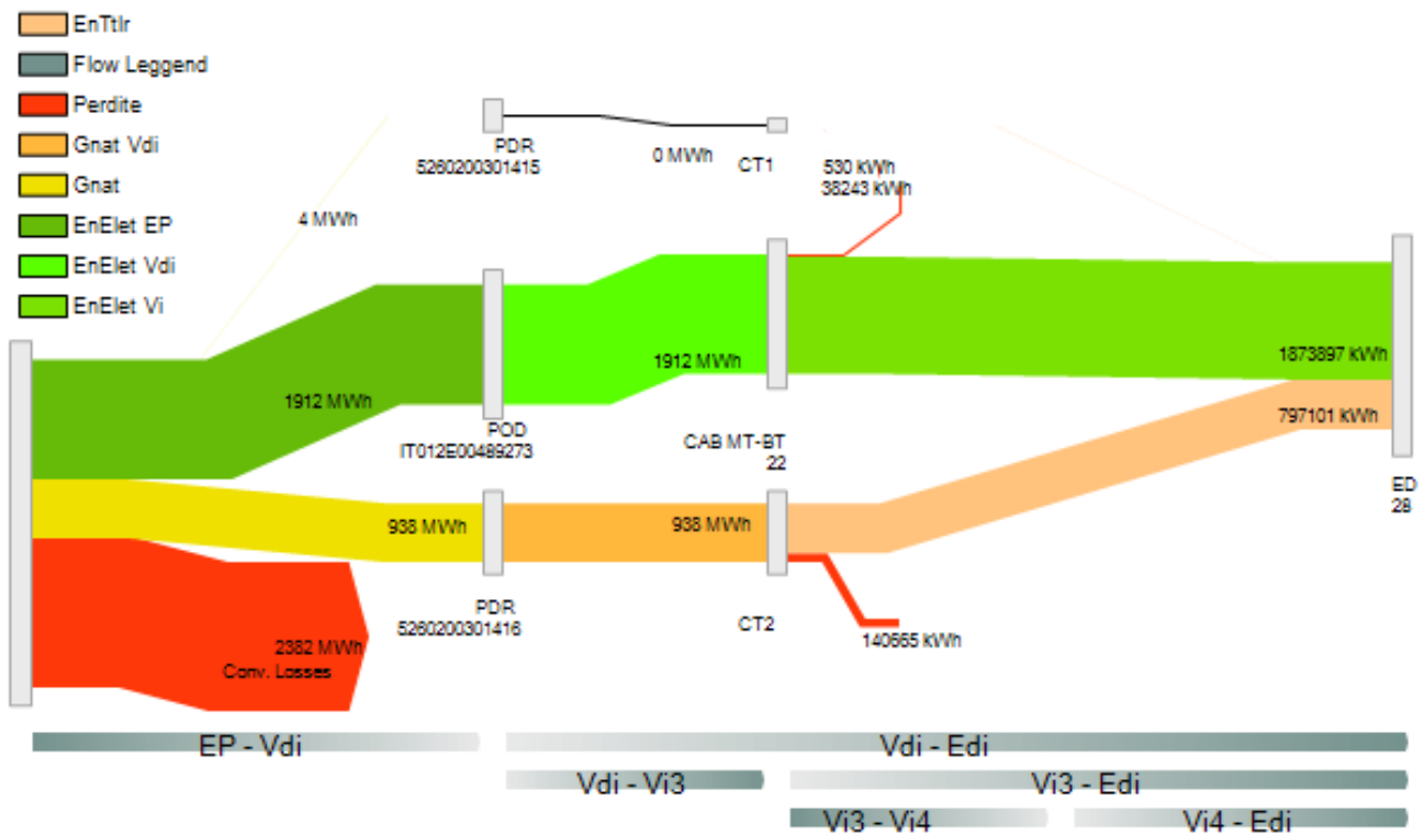
Figura 26. Diagramma di flusso dei vettori energetici, Campus via Mancinelli
