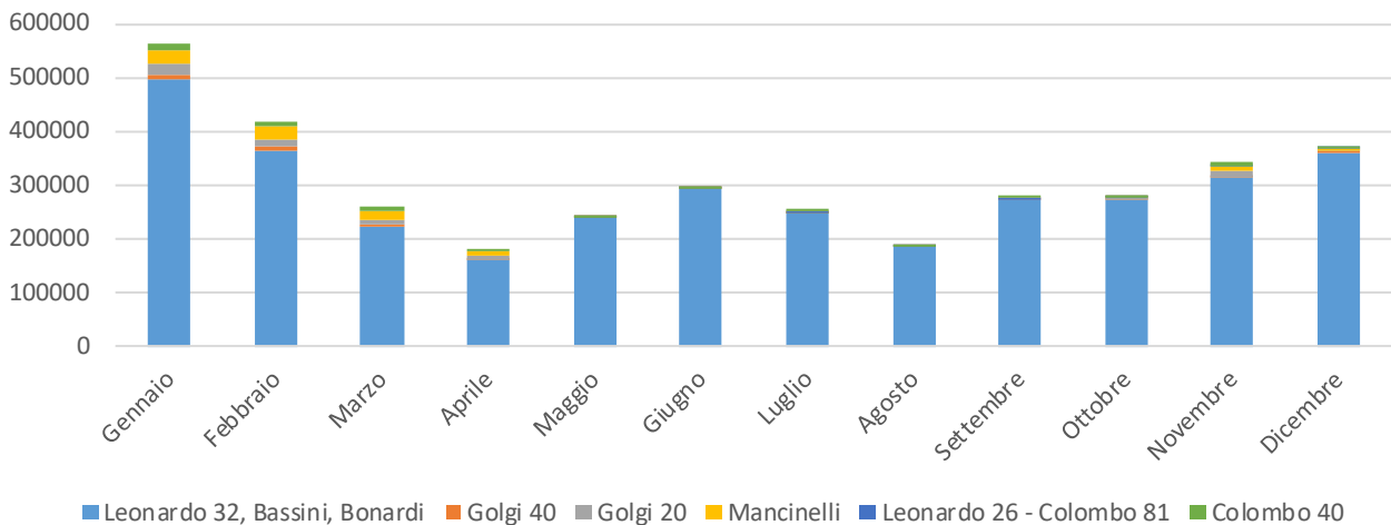
Figura 22. andamento mensile consumo gas naturale [Sm 3 ], Sede Città Studi
