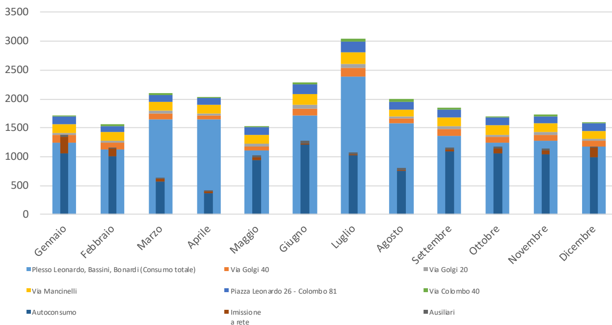
Figura 18. andamento mensile consumo e produzione energia elettrica [MWh], Sede Città Studi
