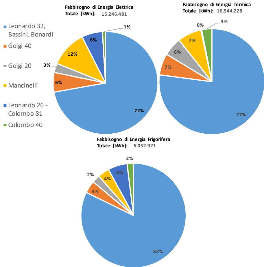
Figura 29. Fabbisogni energetici, Sede Città Studi
