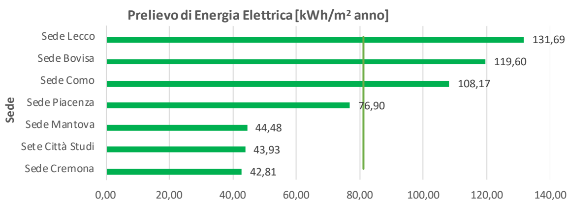
Figura 111. KPI di prelievo Energia Elettrica a livello di Sede
