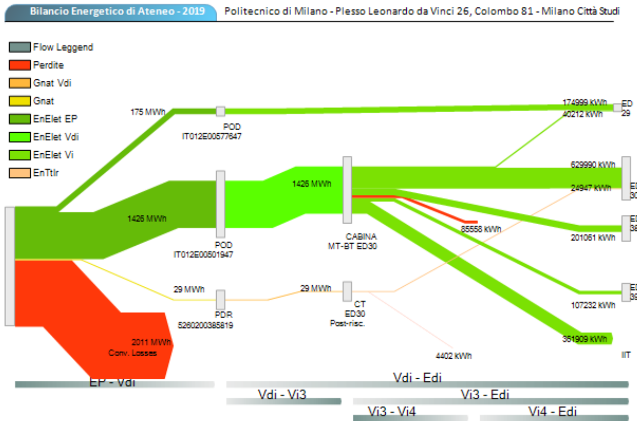
Figura 27. Diagramma di flusso dei vettori energetici, Plesso Leonardo da Vinci 26 - Colombo 81
