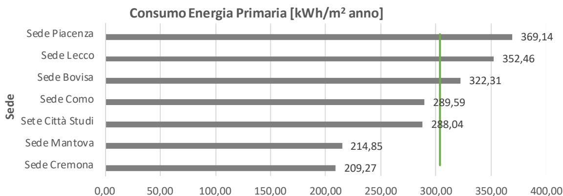
Figura 109. KPI calcolati di consumo Energia Primaria a livello di Sede
