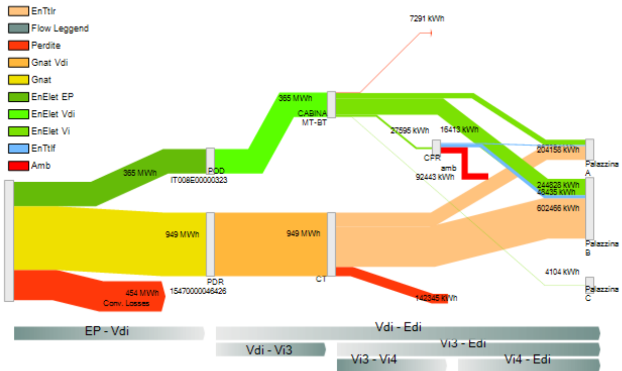
Figura 60. Diagramma di flusso dei vettori energetici, Campus Via Sesto
