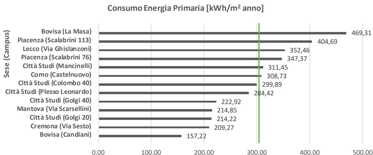
Figura 110. KPI calcolati di consumo Energia Primaria a livello di Campus/Plesso
