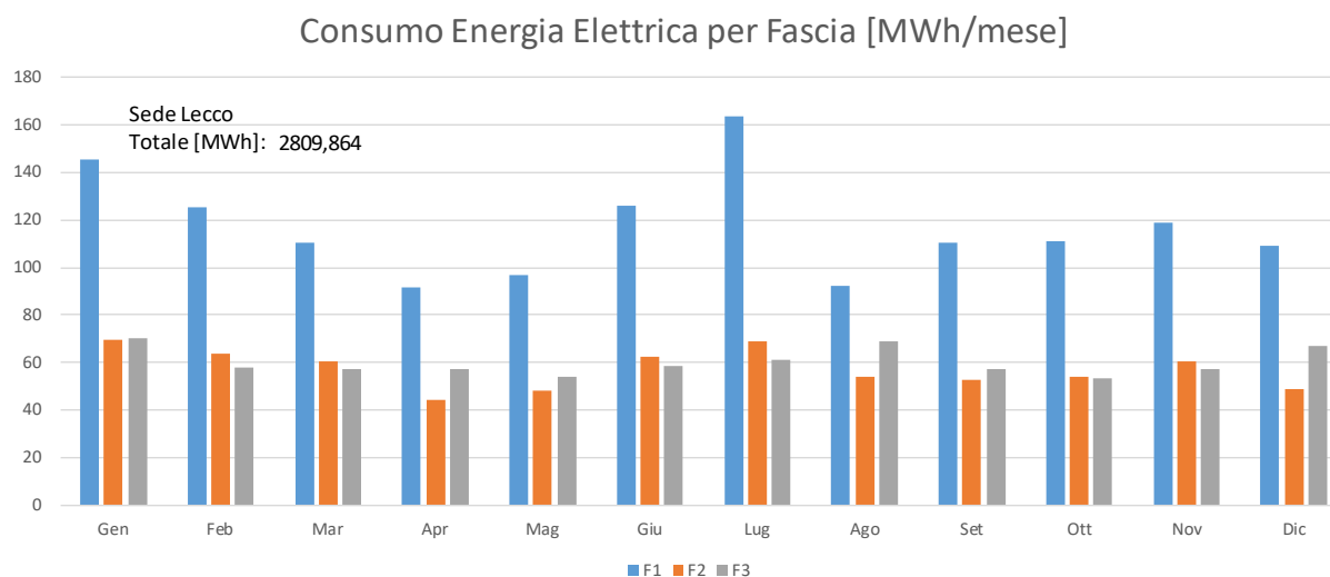
Figura 62. Consumo mensile energia elettrica suddiviso nelle fasce F1, F2, F3, Sede Lecco
