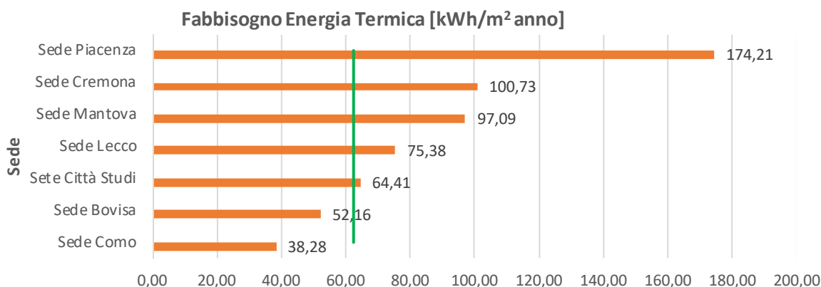
Figura 119. KPI calcolati fabbisogno energia termica a livello di Sede
