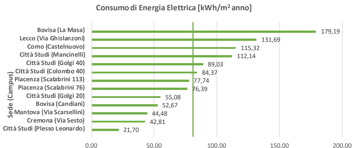
Figura 112. KPI di prelievo Energia Elettrica a livello di Campus
